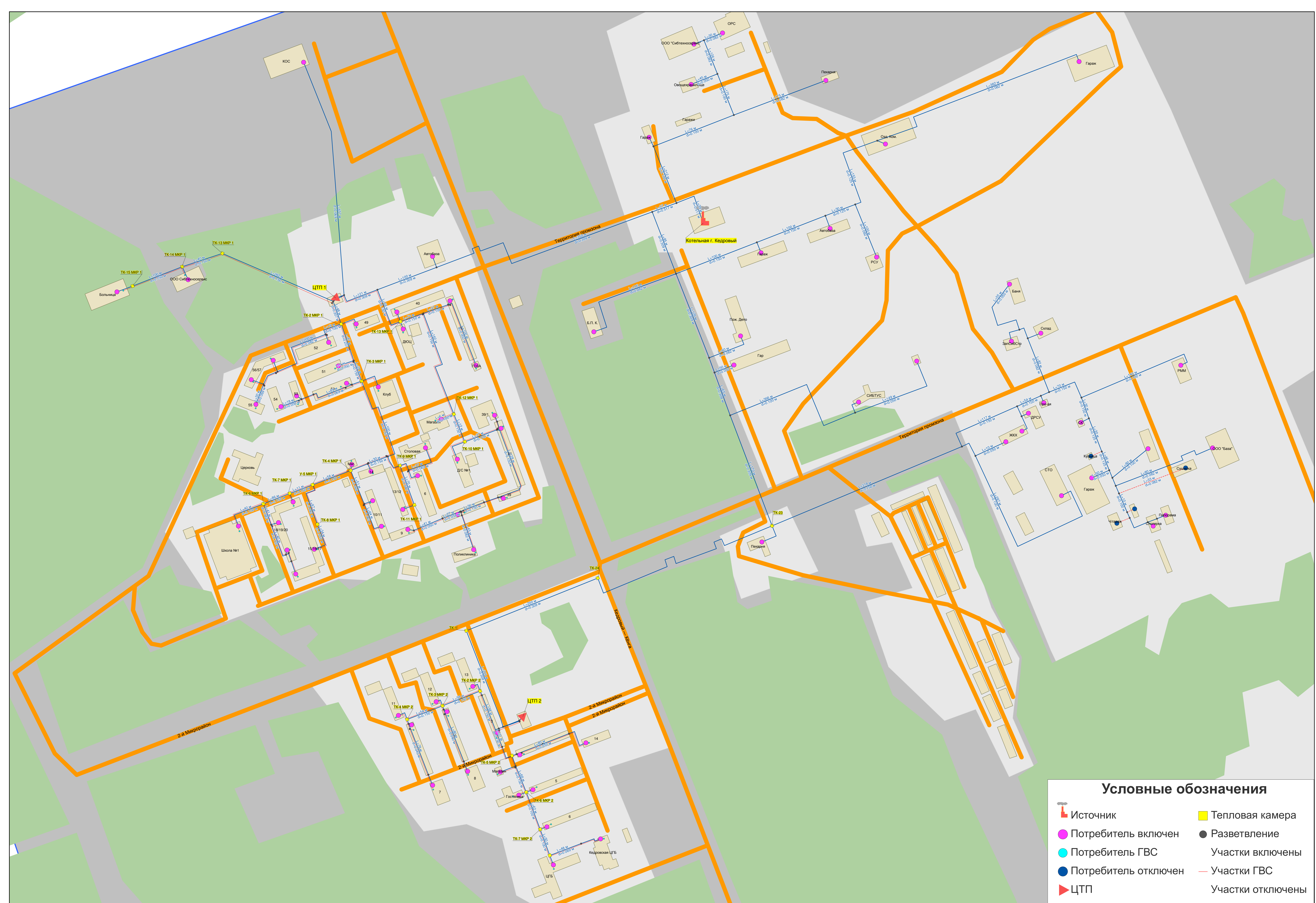
Рис. 1. Схема тепловых сетей Котельной г. Кедровый
